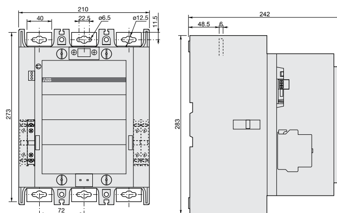
GAF750 AF580, AF750
